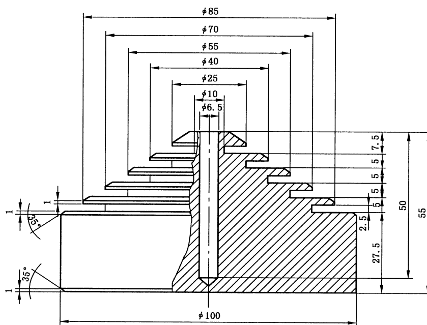
图 1 热源块
